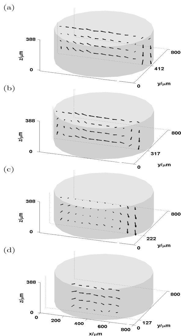
Fig. 7 Slices of x and z velocity components at (a) y = 412 \mu\text{m} ; (b) y = 317 \mu\text{m} ; (c) y = 222 \mu\text{m} ; (d) y = 127 \mu\text{m} .
