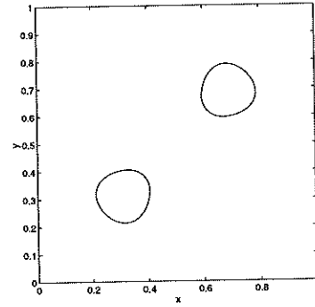
(d) t = 0.03
