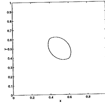
(d) t = 0.0500
