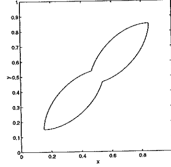
(d) t = 0.1000
